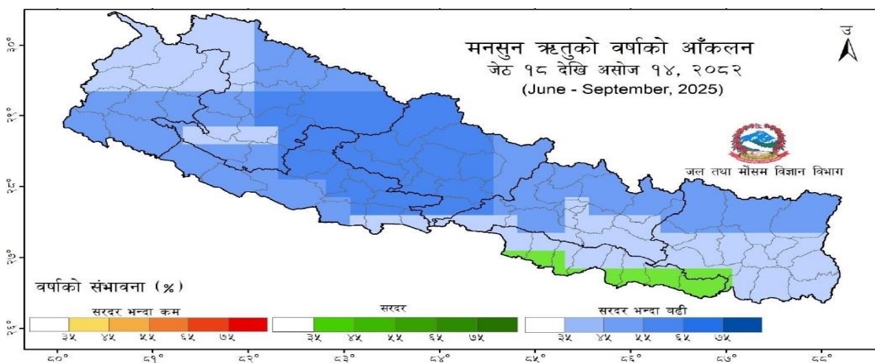
चित्र १: २०८२ को मनसुन ऋतुको वर्षा (सरदर भन्दा कम वा सरदर वा सरदर भन्दा बढी) को सर्वाधिक सम्भावना (highest probability) (%)
