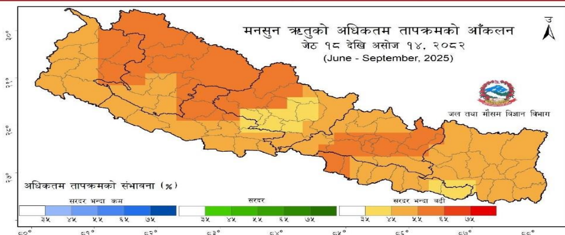
चित्र २: २०८२ को मनसुन ऋतुको अधिकतम तापक्रम (सरदर भन्दा कम वा सरदर वा सरदर भन्दा बढी) को सर्वाधिक सम्भावना (highest probability) (%)
