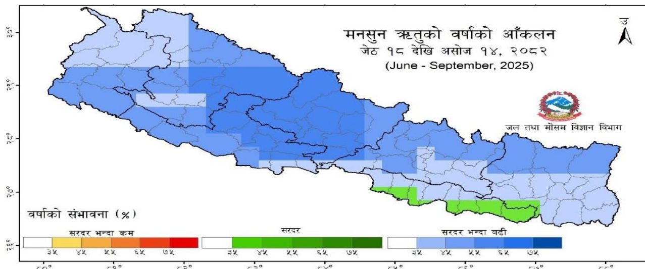
चित्र १: २०८२ को मनसुन ऋतुको वर्षा (सरदर भन्दा कम वा सरदर वा सरदर भन्दा बढी) को सर्वाधिक सम्भावना (highest probability) (%)
